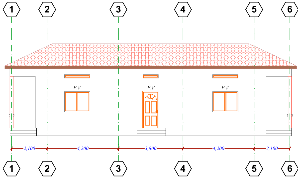
Elevation 01
