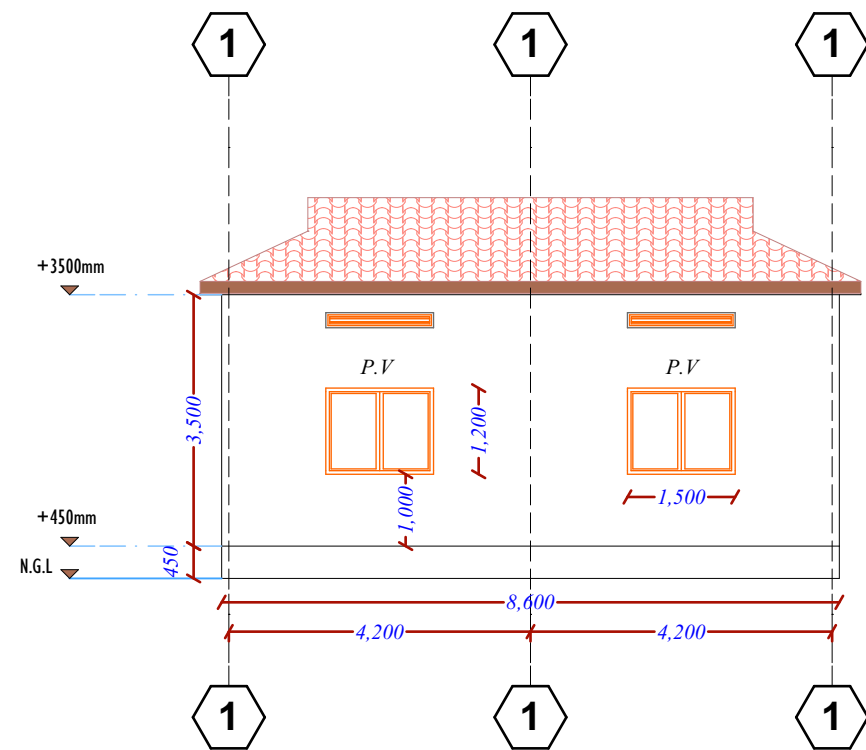
Elevation -03
