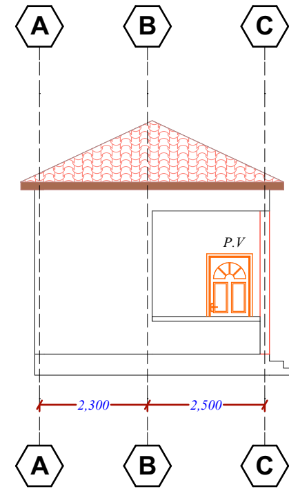
Elevation 02
