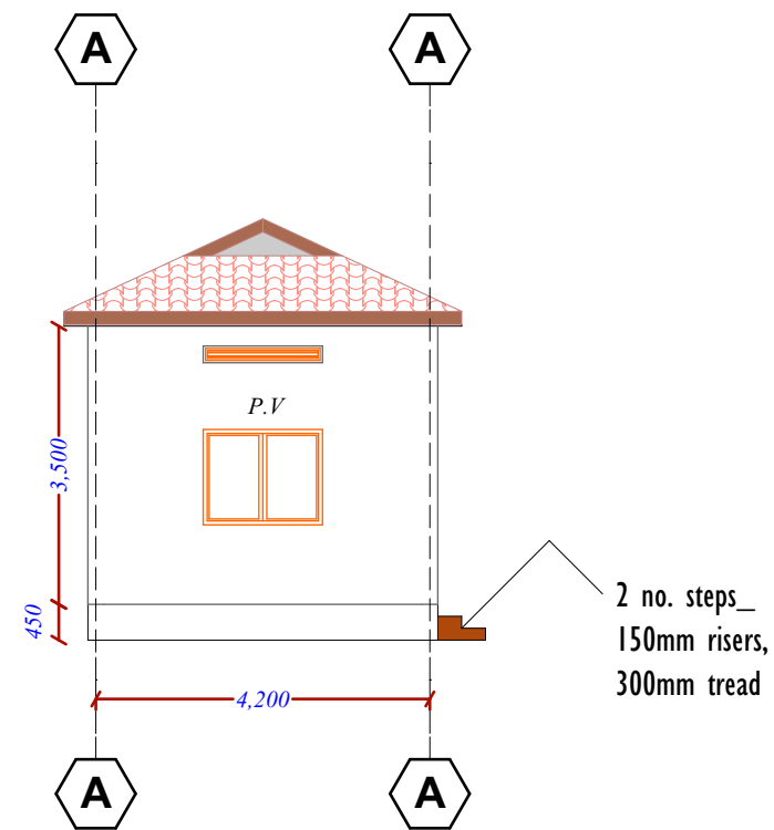
Elevation -04
