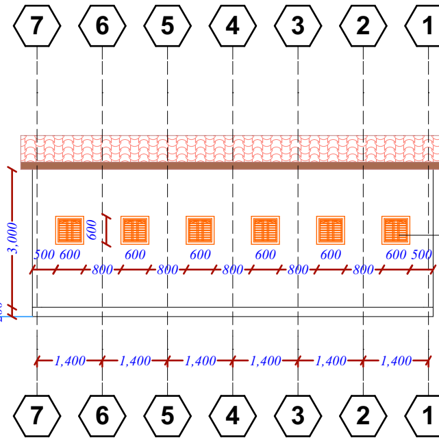
Elevation -03
