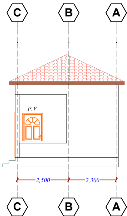
Elevation 04
